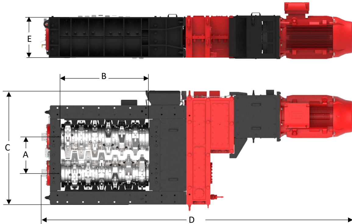
A: Achsabstand | B: Walzenlänge | C: Maschinenbreite | D: Maschinenlänge | E: Maschinenhöhe
